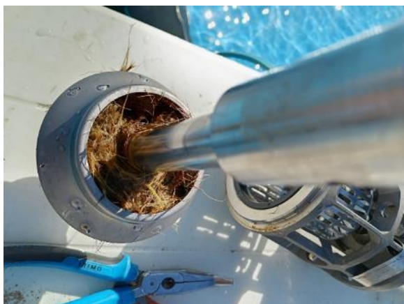
Fuente entrada - Limpieza por acumulación de residuos en tobera cuerpo hidráulico
